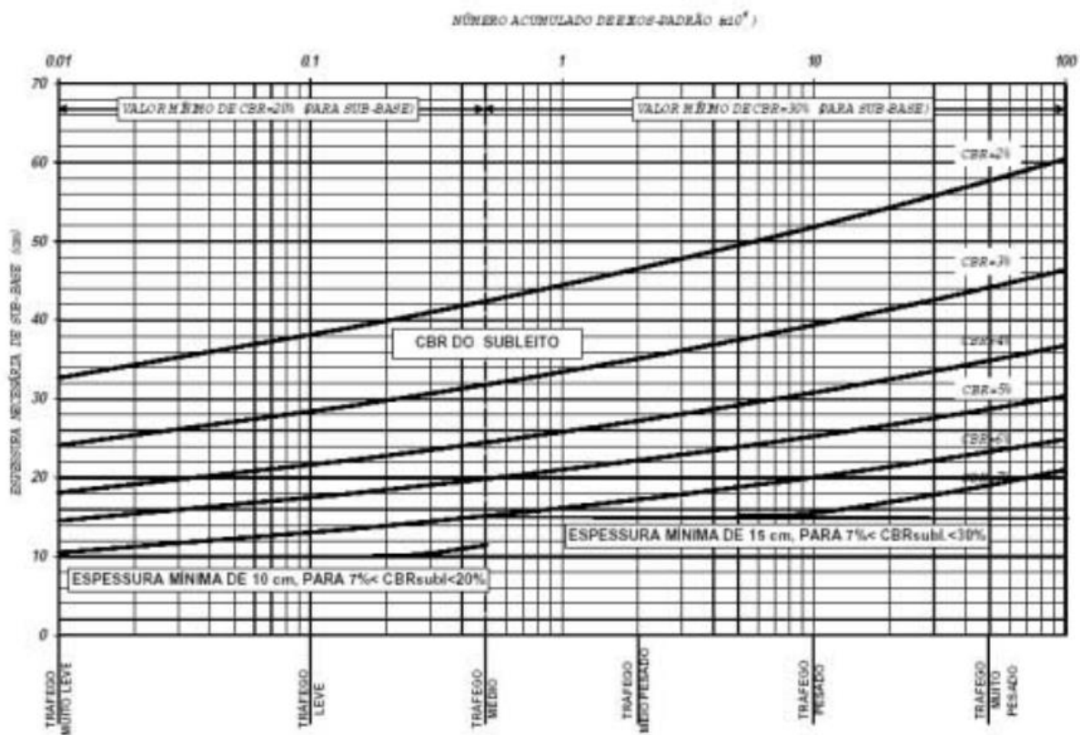
Figura 12 - Espessuras necessárias de sub-base em função do valor de CBR
