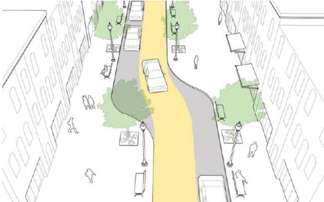
Figura 2 - Ilustração de modelo de chicana (Fonte: NACTO, 2013)
