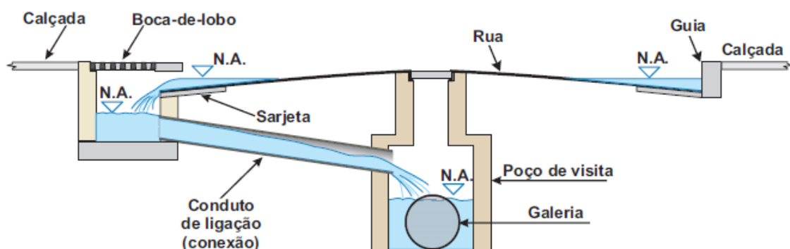
Figura 9 - Poço de visita e demais dispositivos de drenagem para ruas com configuração tradicional.
