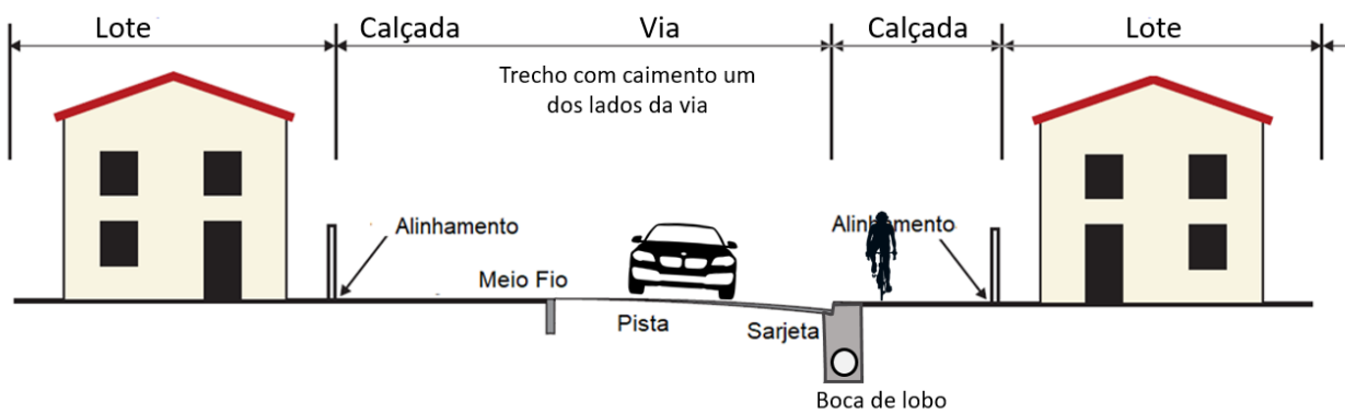
Figura 6 - Exemplo de seção de via com coleta de águas pluviais no eixo
