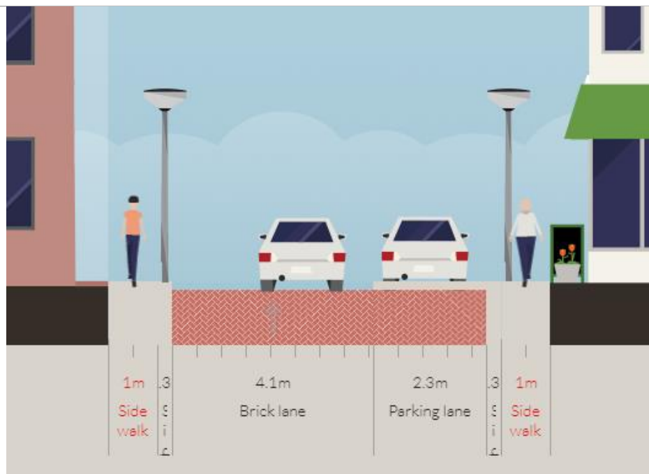
Figura 04: Corte esquemático da seção-tipo atual da rua dos Tabajaras
