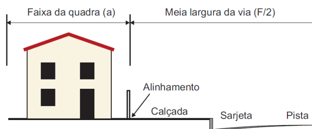
Figura 4 - Exemplo de como se pode considerar as dimensões de uma via com seção convencional. Fonte: Manual De Pavimentação Urbana, Diogo, Francisco José D'almeida, 2008).
