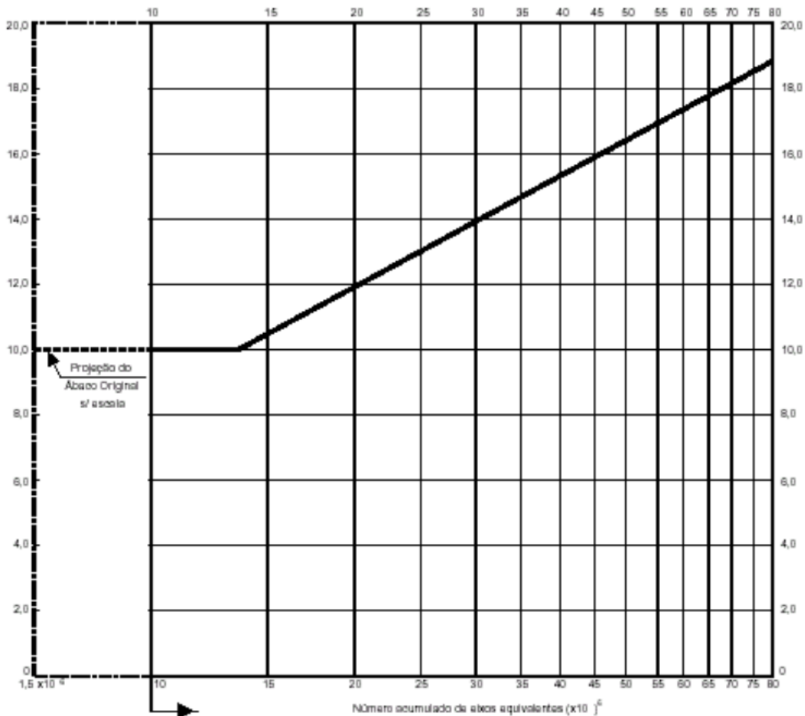
Figura 13 - Espessura da base cimentada em função do número "N"
