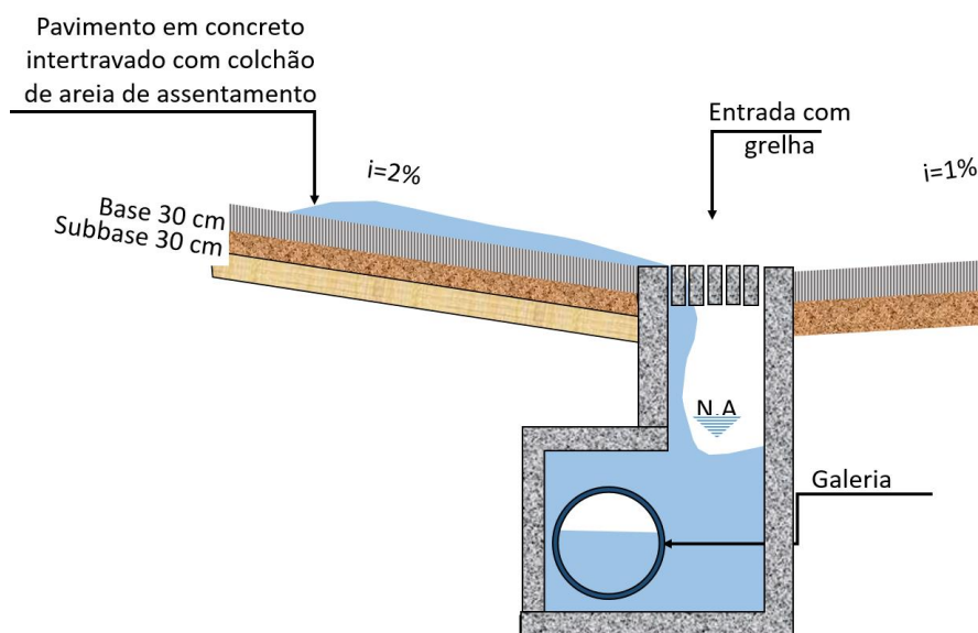
Figura 9 - Poço de visita e demais dispositivos de drenagem para ruas com configuração tradicional.
