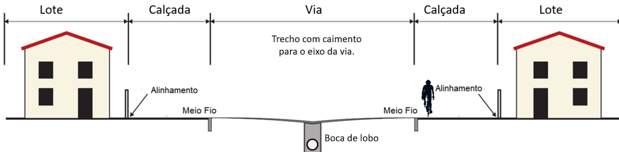
Figura 5- Exemplo de seção de via com coleta de águas pluviais no eixo
